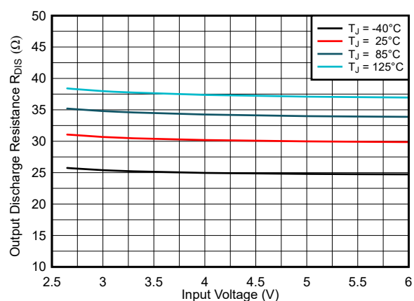
図 6-4. Discharge Resistance
