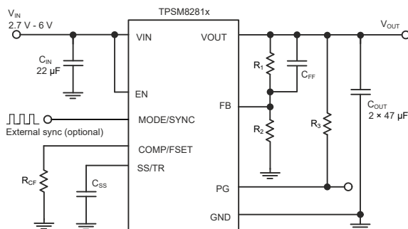
回路図
