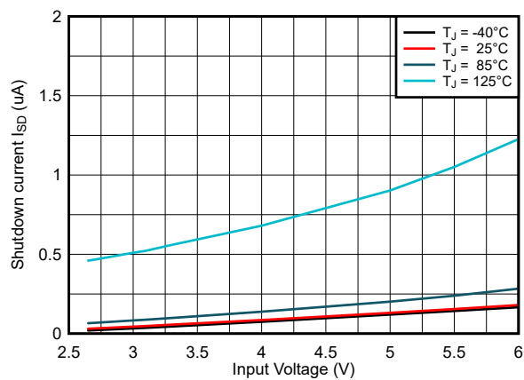
図 6-2. Shutdown Current
