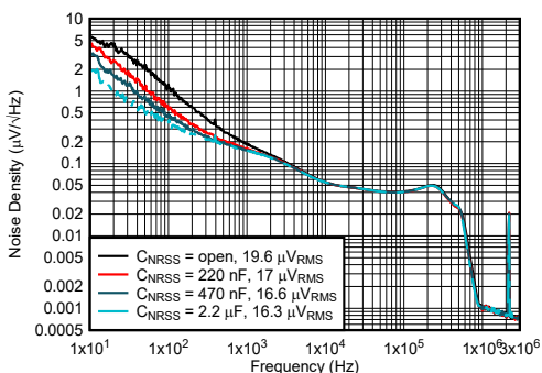
出力ノイズと周波数との関係
