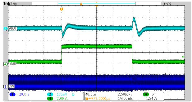
8-9. Load Transient
