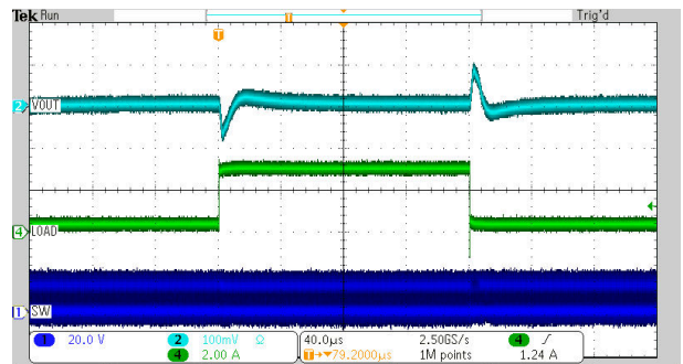
8-11. Load Transient
