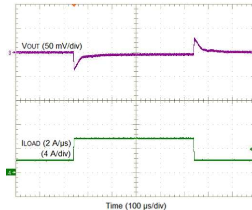
図 16. V_{OUT} = 0.8\text{ V} , 4-A Load Step
