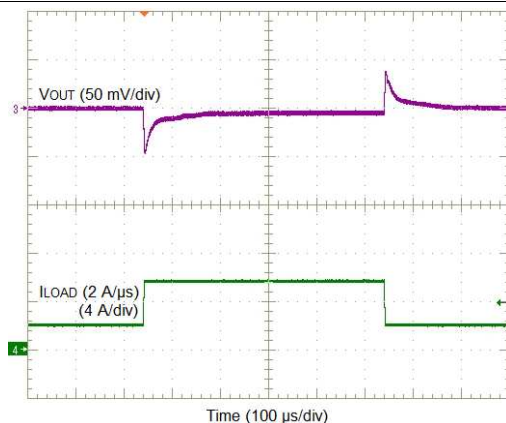
図 17. V_{OUT} = 1\text{ V} , 4-A Load Step
