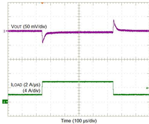
図 15. V_{OUT} = 0.8\text{ V} , 4-A Load Step
