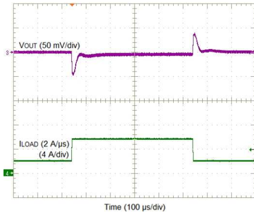
図 15. V_{OUT} = 0.8\text{ V} , 4-A Load Step
