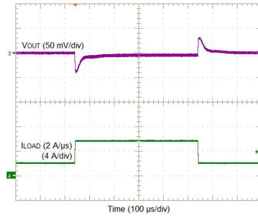
図 16. V_{OUT} = 0.8\text{ V} , 4-A Load Step
