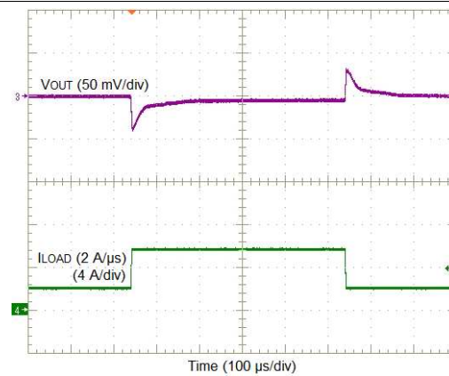
図 18. V_{OUT} = 1\text{ V} , 4-A Load Step
