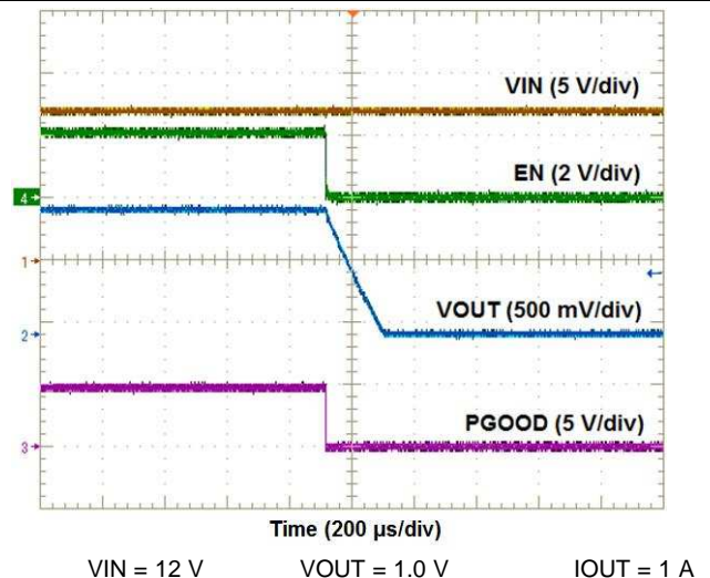
⊗ 10. EN Shut-down Waveforms
