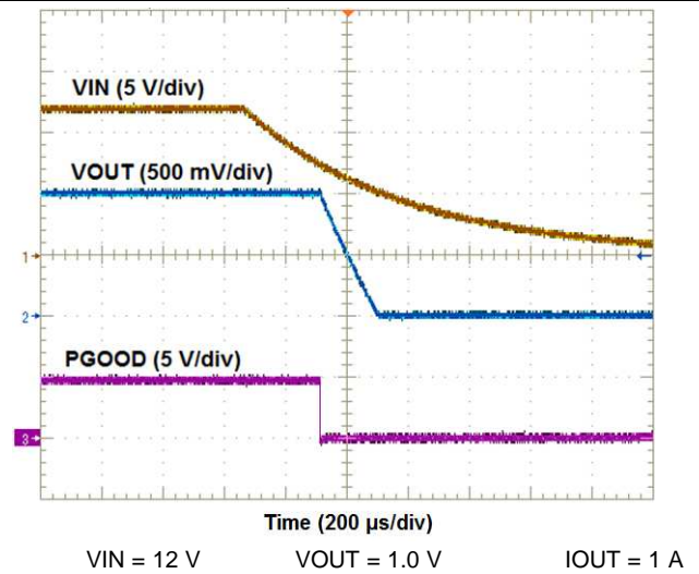
⊗ 8. VIN Shut-down Waveforms
