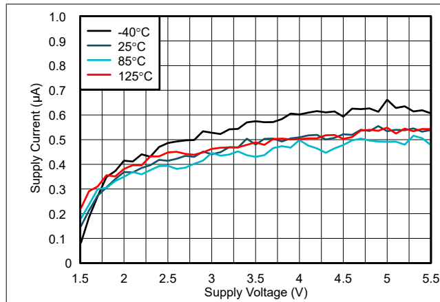
図 5-2. 電源電流と電源電圧との関係
