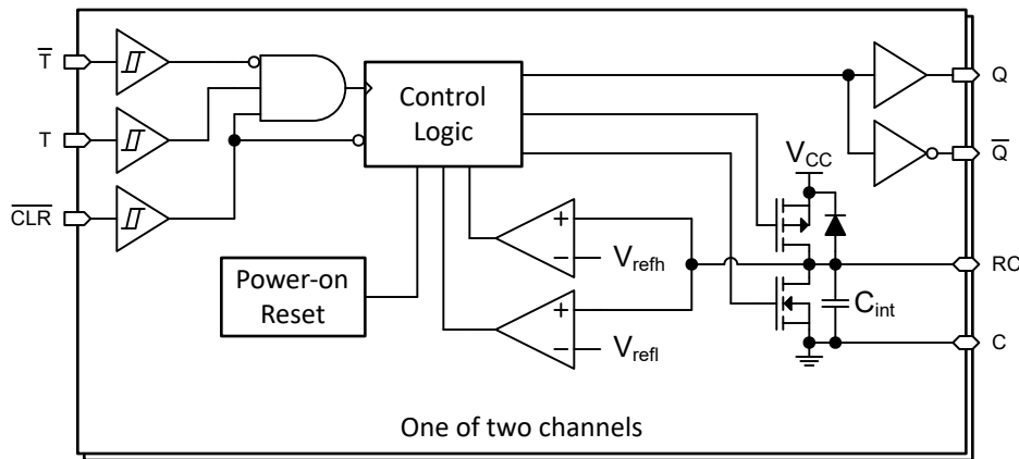
図 7-3. TPUL2G122-Q1
