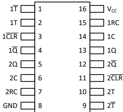
図 4-1. TPUL2G122-Q1 D および PW パッケージ 16 ピン SOIC および TSSOP 上面図 図 4-2. TPUL2G122A-Q1 D および PW パッケージ 16 ピン SOIC および TSSOP 上面図
