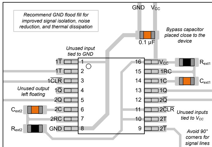
図 8-6. PW (TSSOP) パッケージの TPUL2G122x-Q1 のプッシュプルレイアウト例
