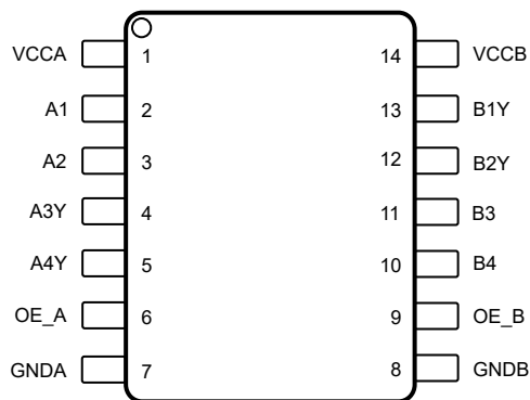
図 4-4. TXGx042DYY 14 ピン SOT 上メンス
