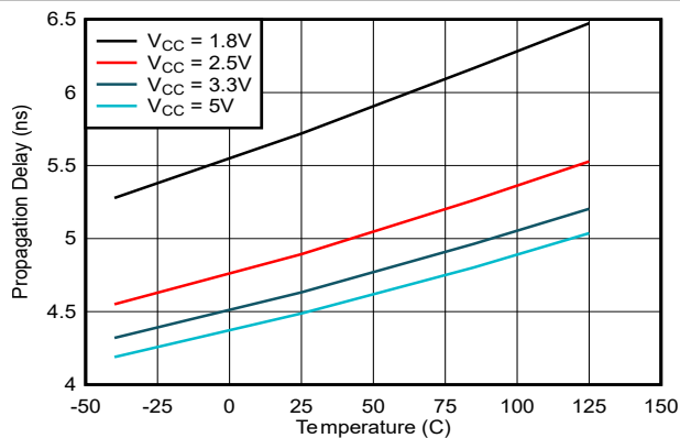
図 5-6. 伝搬遅延、 T_{PHL} 、と温度との関係
