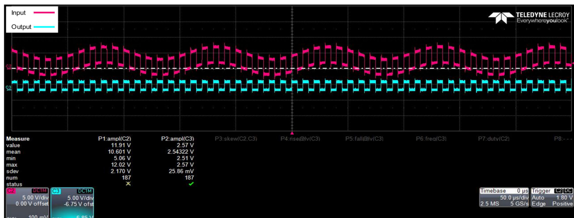
図 7-5. 10kHz における AC グランドノイズ 2V pp による 5V から 2.5V への I/O 変換を示す波形
