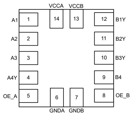
図 4-1. TXGx041 RUC パッケージ 14 ピン X2QFN 上面図
