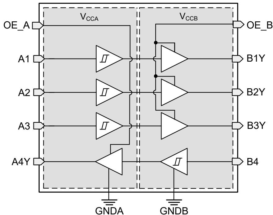
図 7-1. TXG1041 の機能ブロック図
