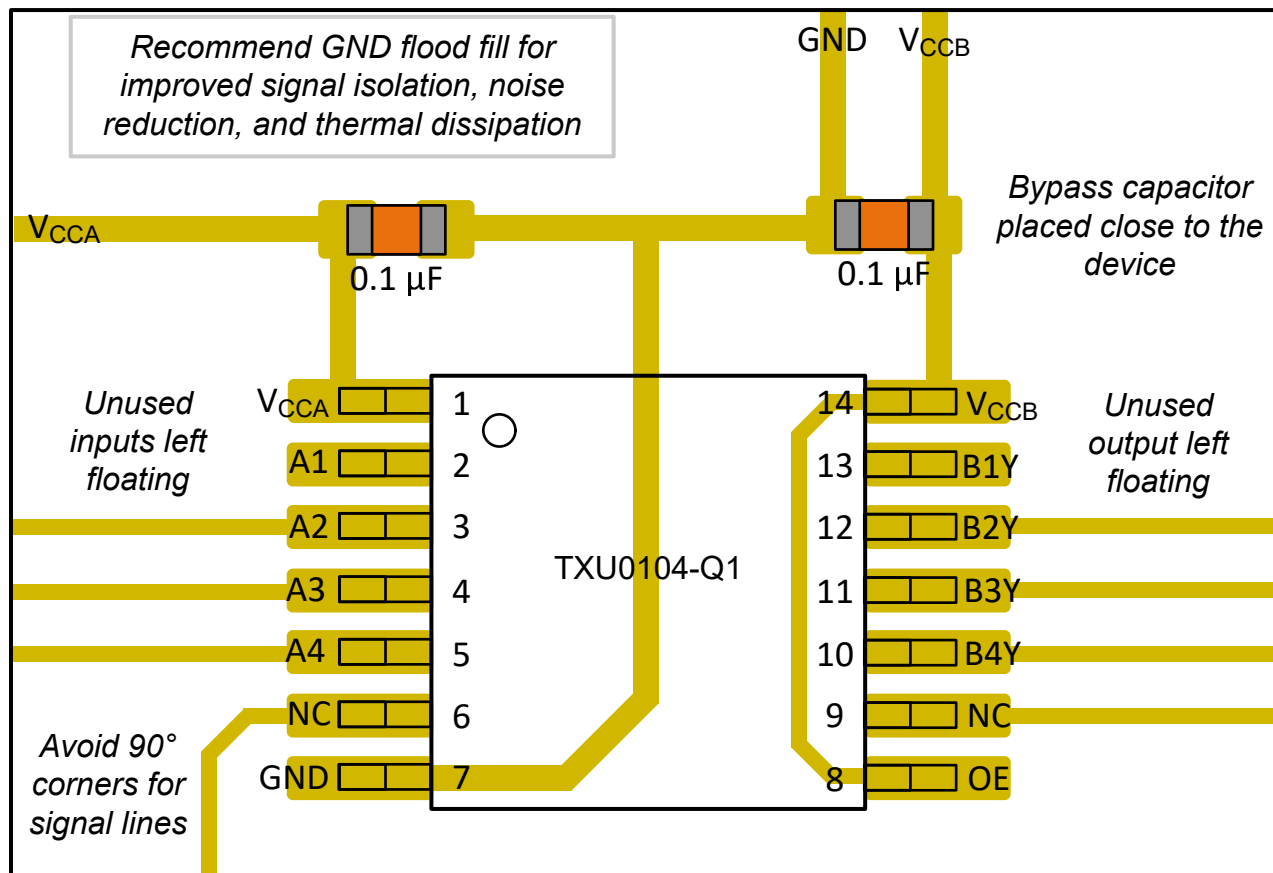
✎ 12-1. Layout Example – TXU0104-Q1
