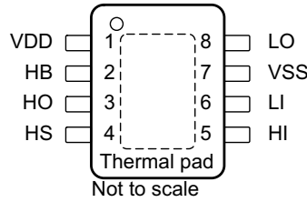
図 4-1. DDA パッケージ 8 ピン SO-PowerPAD 上面図
