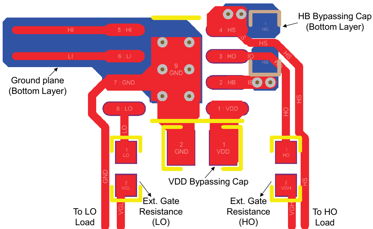
図 9-1. UCC27212A-Q1 のレイアウト例
