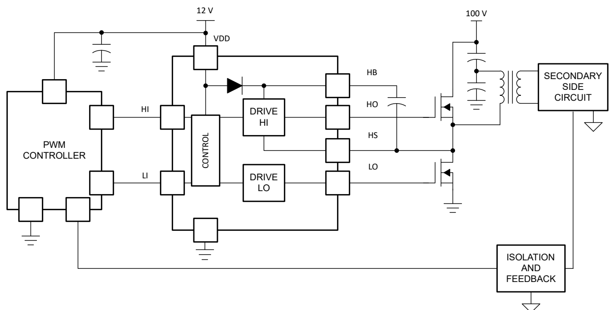
図 7-1. UCC27212A-Q1 の代表的なアプリケーション
