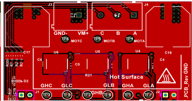
☒ 5-7. Bottom Layer
