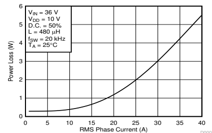
電力損失と出力電流との関係
