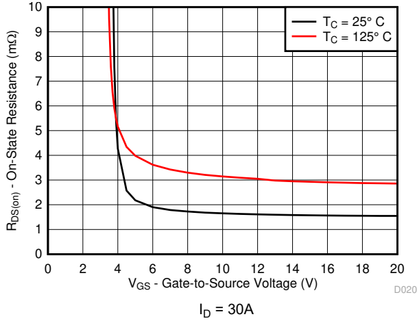
4-13. MOSFET R_{DS(on)} vs V_{GS}
