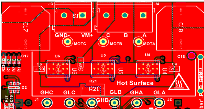
☒ 5-6. Top Layer
