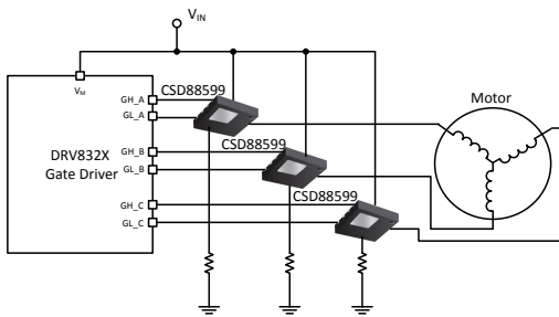
回路例
