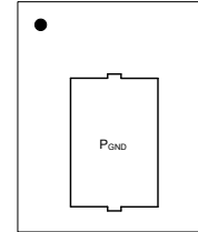
上面図
