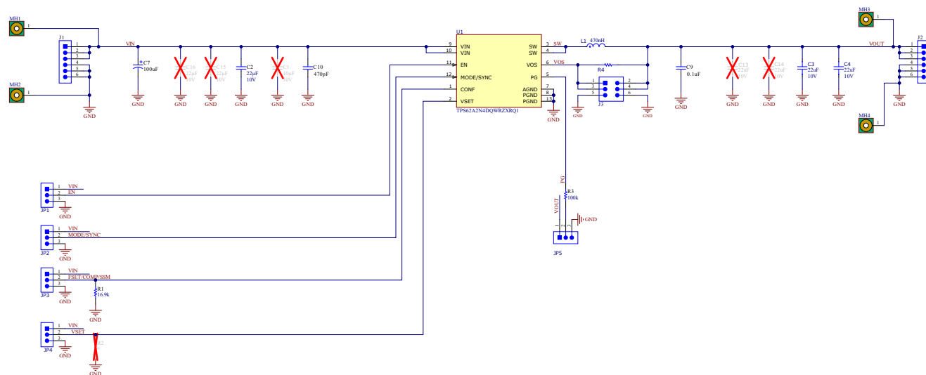
図 3-1. TPS62A204QEVM-116 の回路図
