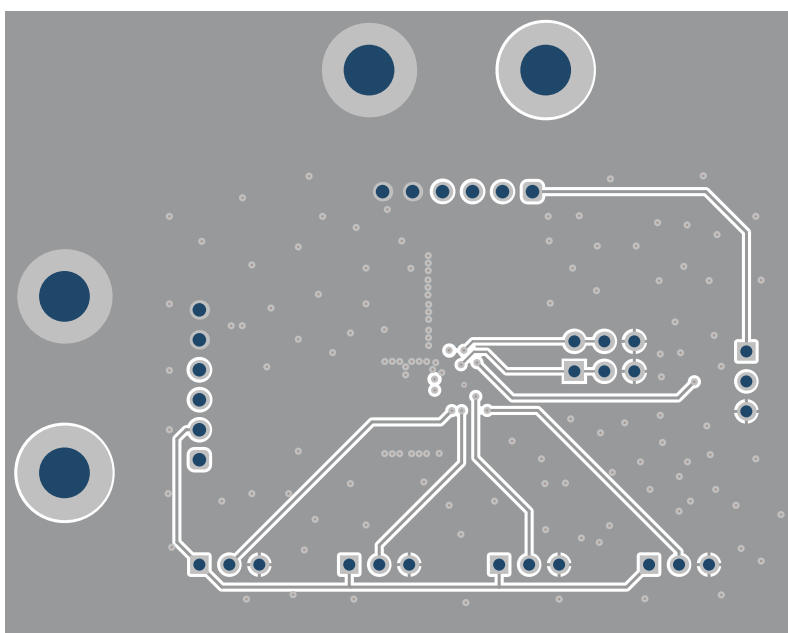
図 3-5. 信号層 2
