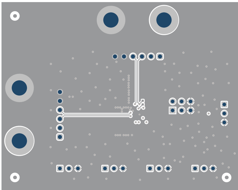
図 3-6. 下層
