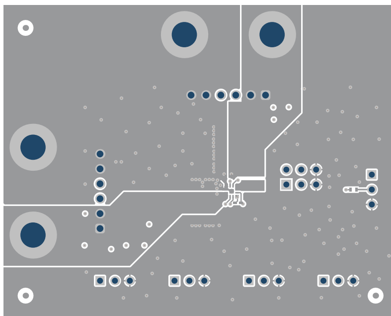
図 3-3. 上層
