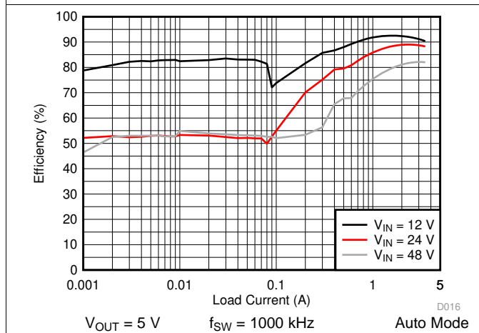
图 27. LM76003 Efficiency
