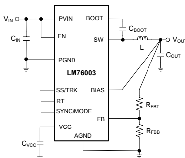
概略回路図
