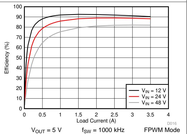
图 28. LM76003 Efficiency
