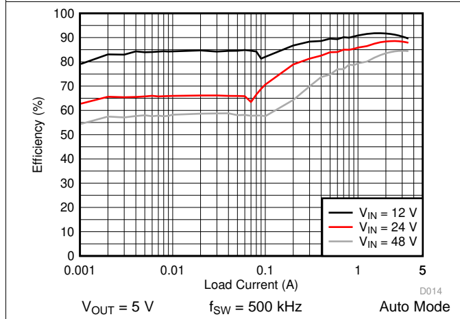
图 25. LM76003 Efficiency
