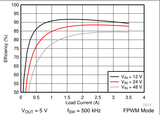
图 26. LM76003 Efficiency
