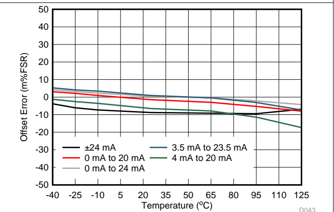
图 47. IOUT Offset Error vs Temperature
