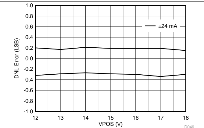
图 51. IOUT Bipolar Range DNL vs VPOS
