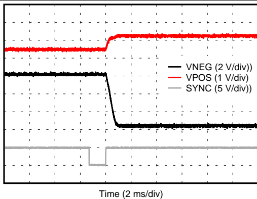
78. VPOS & VNEG Enable Settling Time
