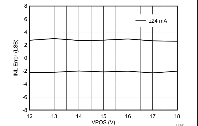
图 49. IOUT Bipolar Range INL vs VPOS
