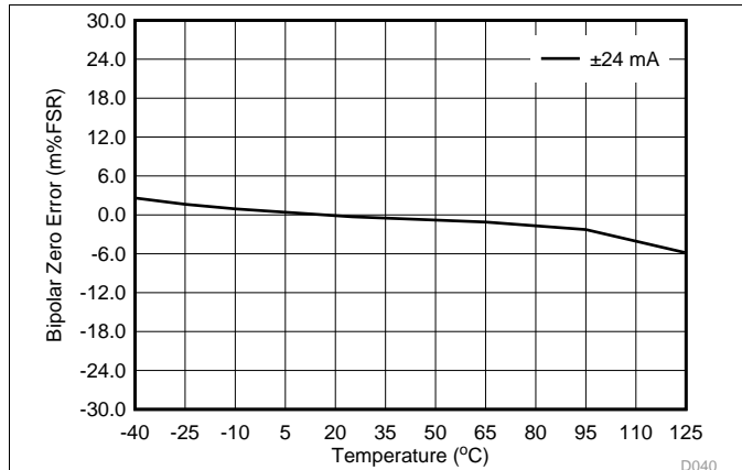
图 44. IOUT Bipolar Zero Error vs Temperature
