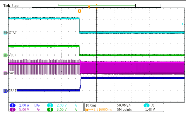
10-9. Charge Enable
