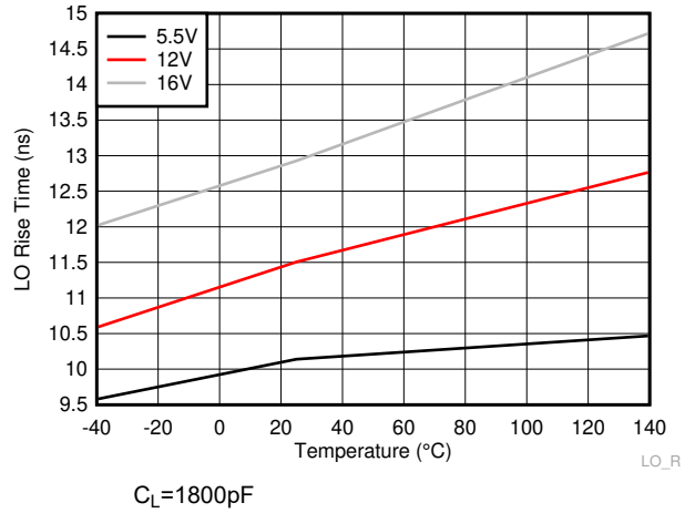
6-22. LO Rise Time
