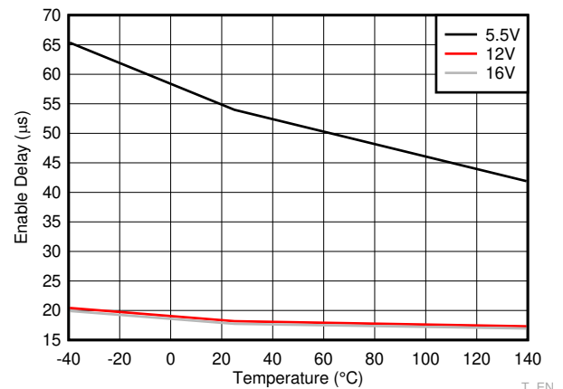
6-12. Enable Delay
