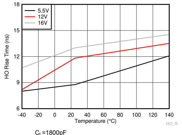
6-24. HO Rise Time
