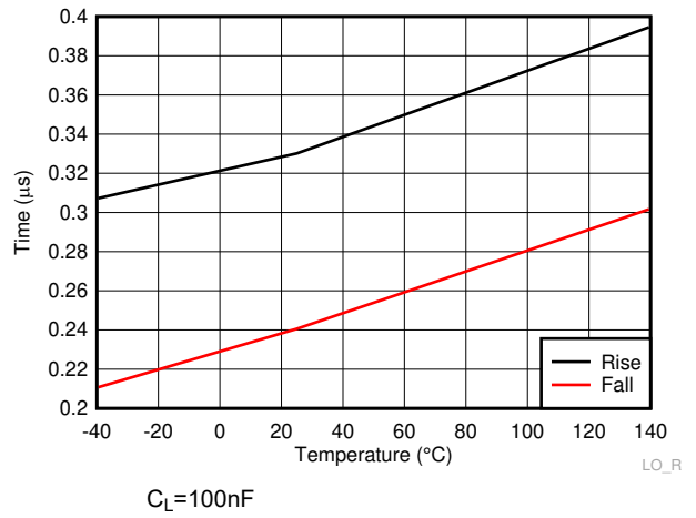
6-26. LO Rise & Fall Time
