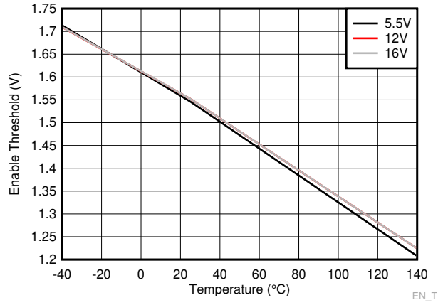
6-10. Enable Threshold
