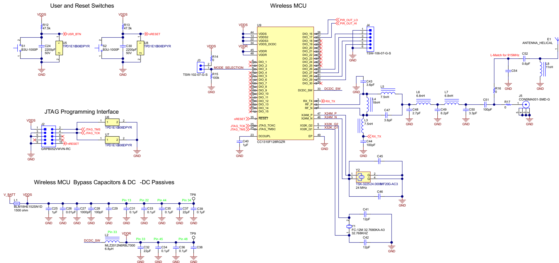
25. Wireless MCU Schematic
