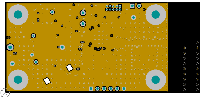
図 29. GND Layer
