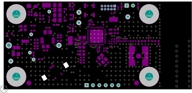
図 27. Top Solder Mask
