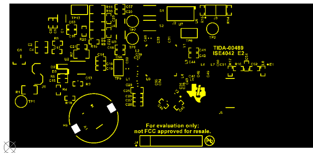
図 26. Top Silkscreen
