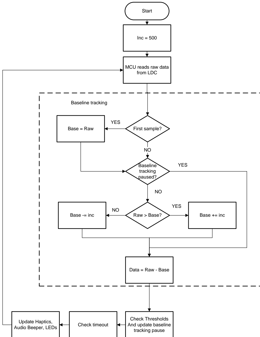
図 18. Baseline Tracking
