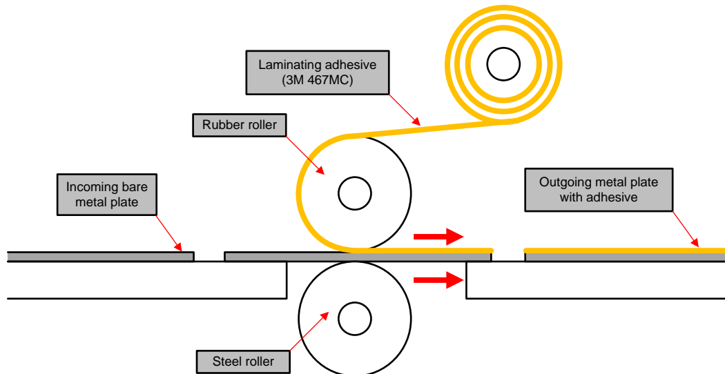
図 23. Lamination Technique
