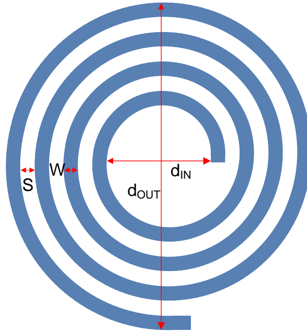
図 11. PCB Coil Parameters
