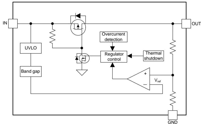
図 4. TPS7B6933-Q1 Functional Block Diagram
