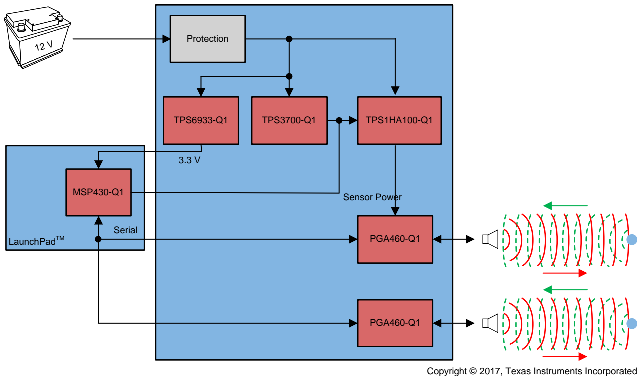
図 1. TIDA-01424 Block Diagram
