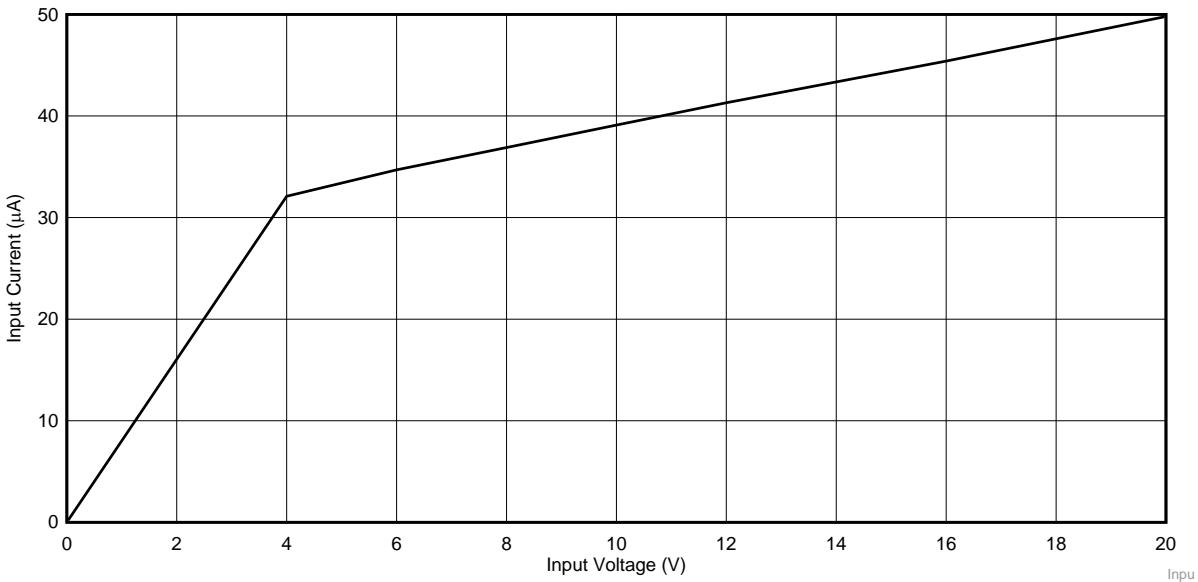
Input Current vs Voltage Standby.grf
