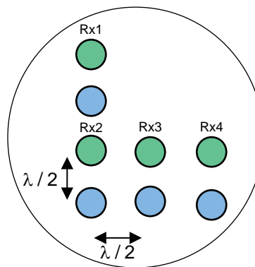
図 7. Angle Spectrum
