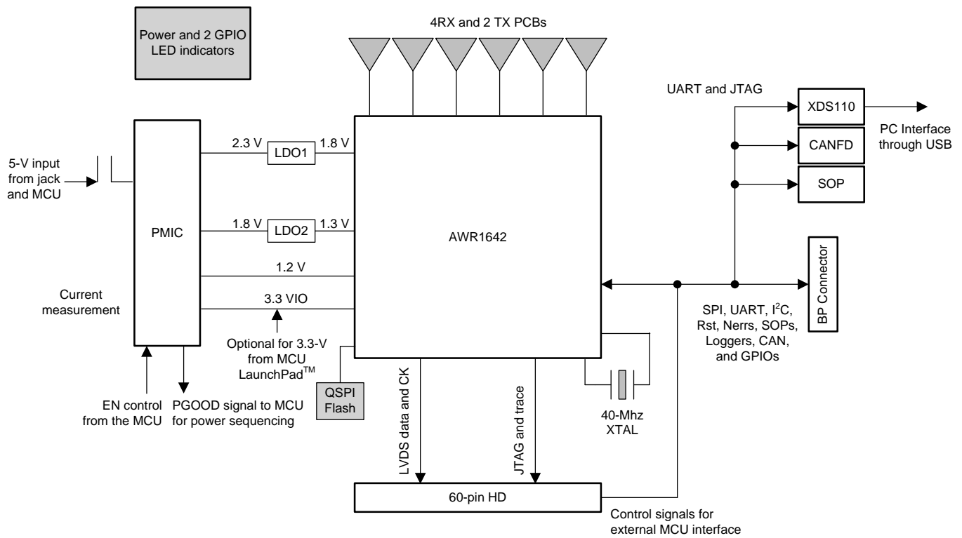
図 2. AWR1642 EVM Block Diagram
