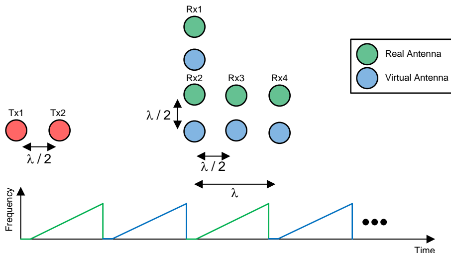
図 3. ODS EVM-Antenna Configuration
