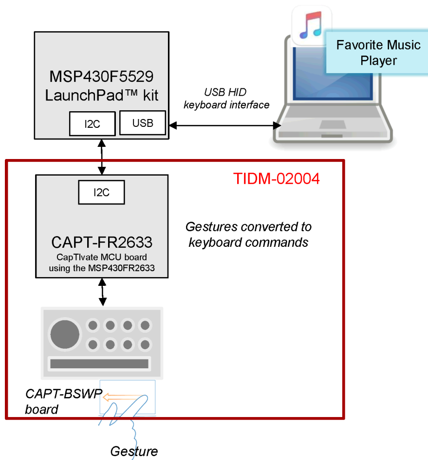
図 1. TIDM-02004 Block Diagram
