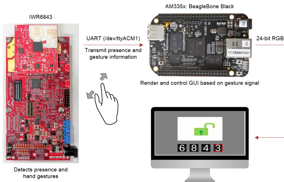
図 3. TIDEP-01013 Block Diagram
