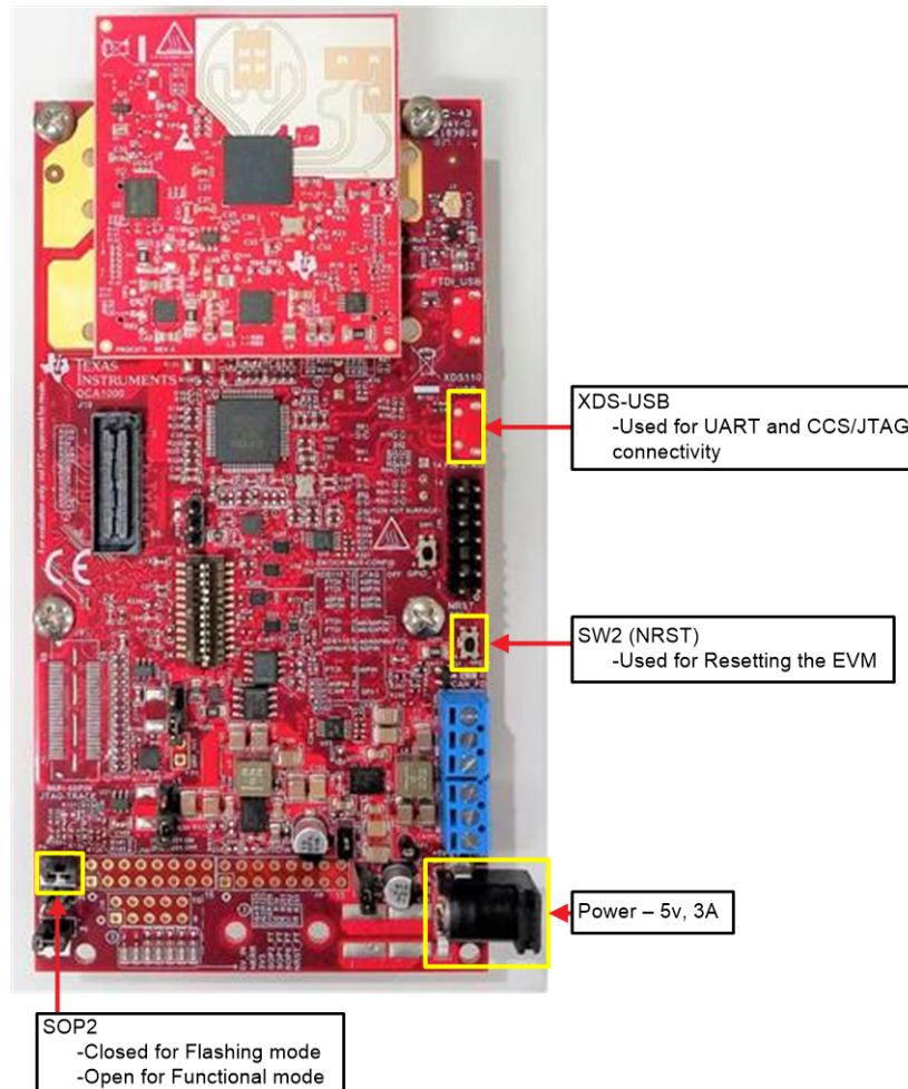
図 7. mmWave EVM Orientation
