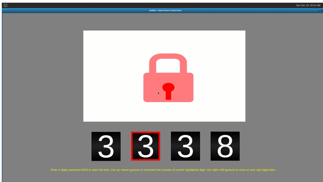
図 10. Left-Swipe Gesture
