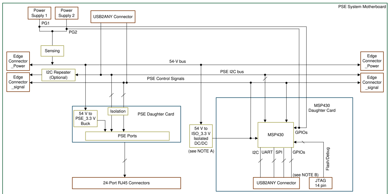
図 1. TIDA-050026-23881 Block Diagram
