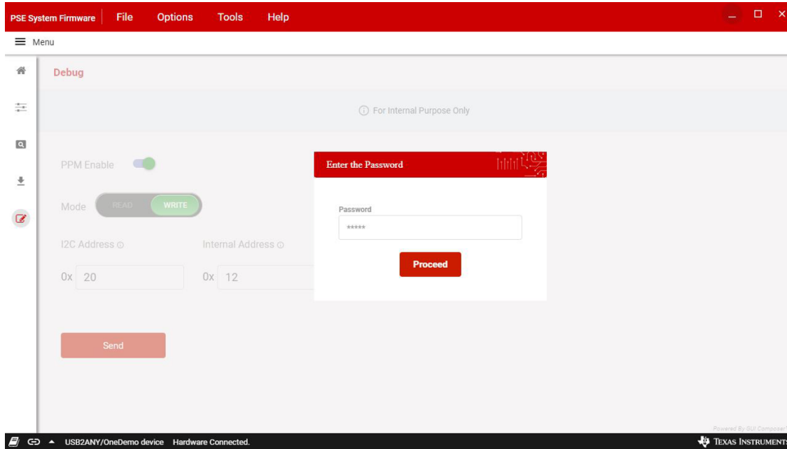
図 16. Debug Page
