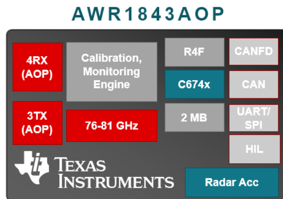
図 2-3. AWR1843AOP Block Diagram
