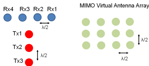
図 2-4. AWR1843AOP Antenna Virtual Array
