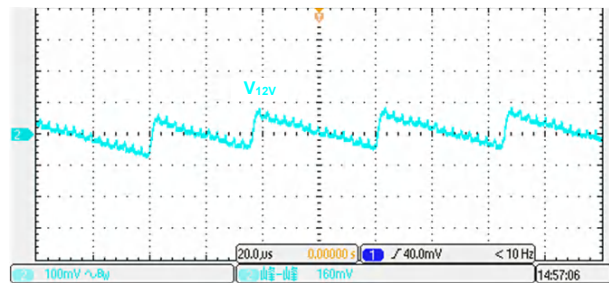
図 3-5. 12-V Ripple
