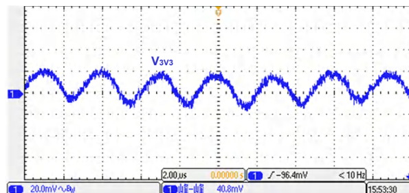
図 3-6. 3.3-V Ripple
