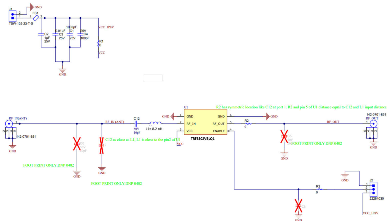
図 3-1. L1 バンドの TRF3302Q1EVM 回路図
