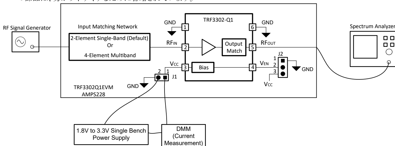
図 2-1. ゲインと出力 P1dB を目的とした TRF3302Q1EVM 向けシングルトーン設定
