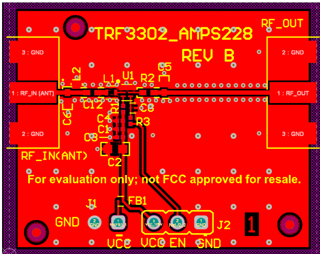
図 3-4. 上層
