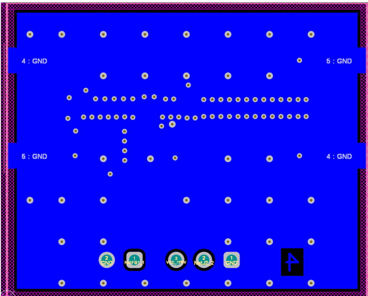
図 3-7. 下層
