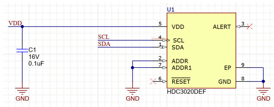
図 2-1. HDC3020FLXEVM の回路図
