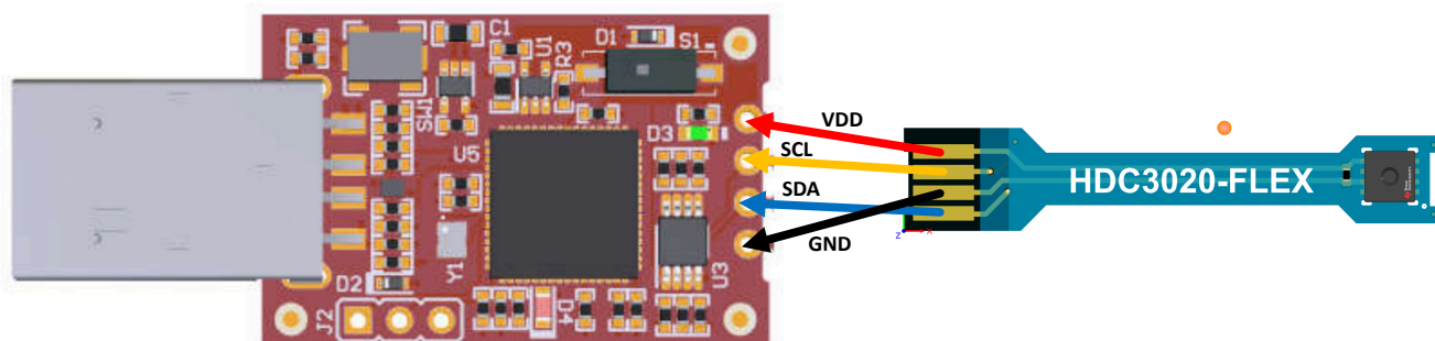
図 1-3. HDC3020FLXEVM の HDC3020EVM への半田付け
