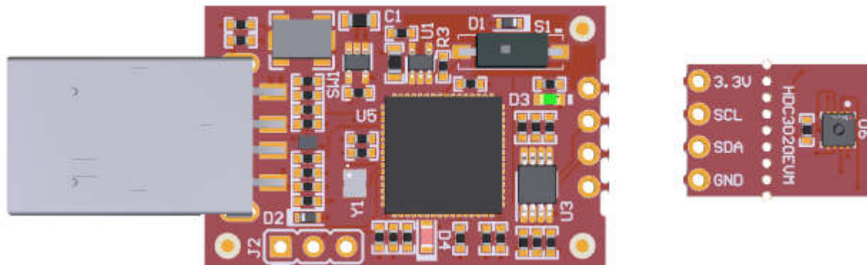
図 1-2. HDC3020EVM の切り離し可能セクション
