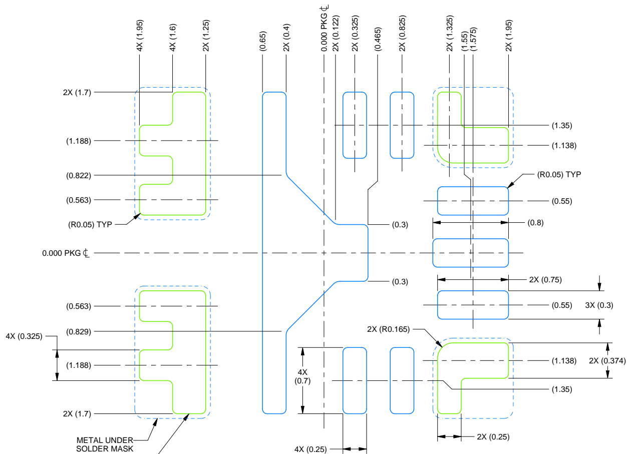
LAND PATTERN EXAMPLE SCALE: 25X
