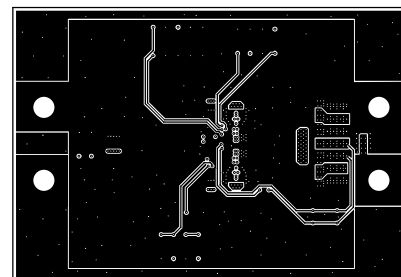
Figure 4-9. Layer 7
