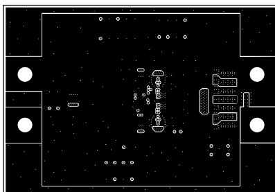
Figure 4-8. Layer 6
