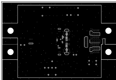
Figure 4-6. Layer 4
