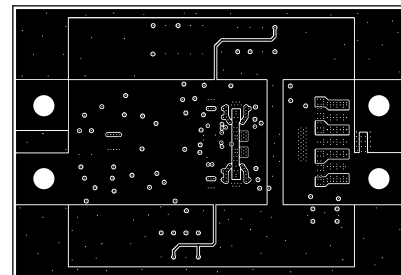
Figure 4-7. Layer 5
