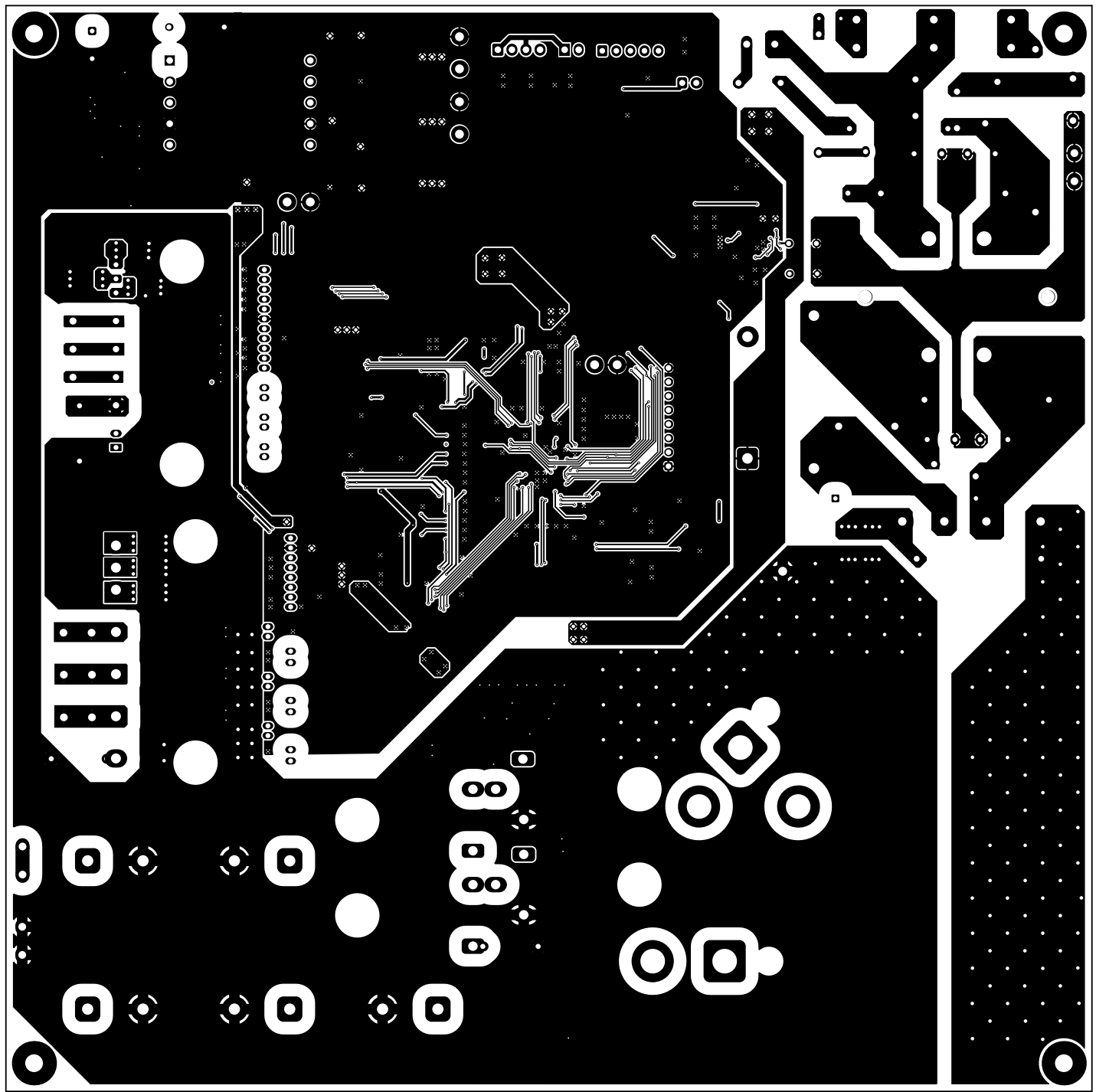
Bottom Layer
