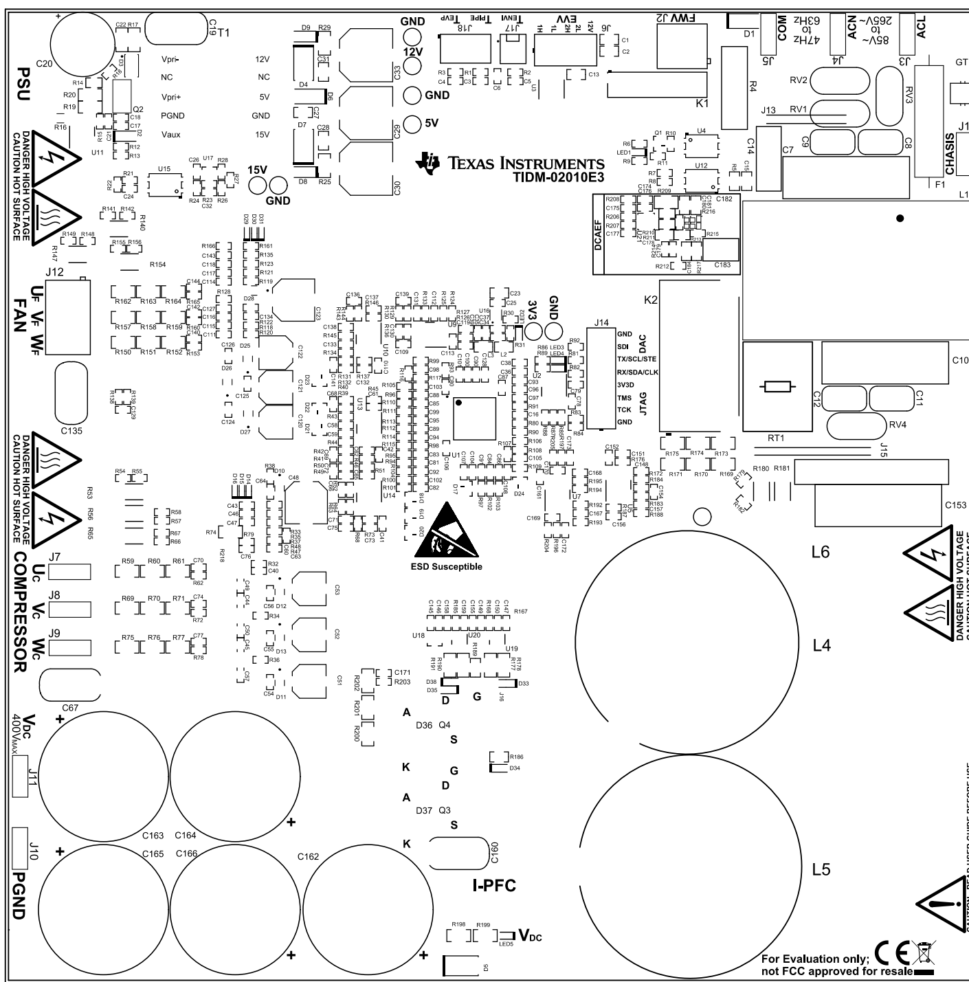
Top Overlay
