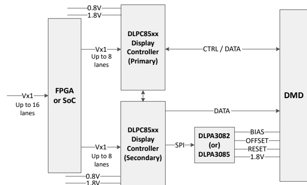
4K UHD Display Chipset
