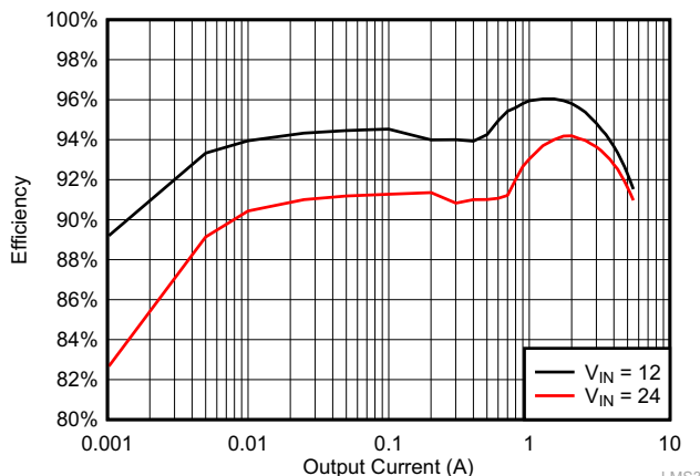
LMS3655-Q1 Efficiency: V_{OUT} = 5\text{ V}
