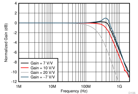
V_{OUT} = 2\text{ V}_{PP}
