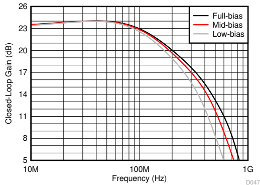
A_V = 15\text{ V/V} , V_O = 16\text{ V}_{PP}
