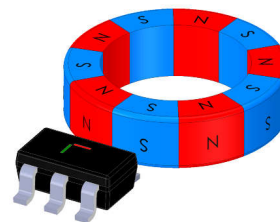
Figure 7-6. XY Outer Edge 2
