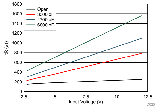
Different C_{dV/dt} values D025
