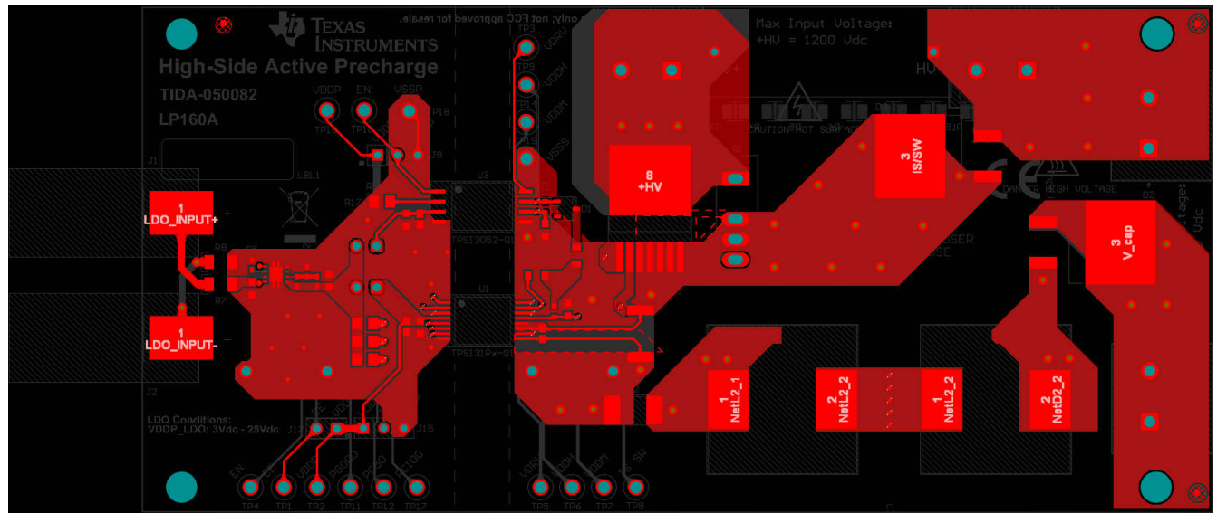
Figure 7-6. Top Layer
