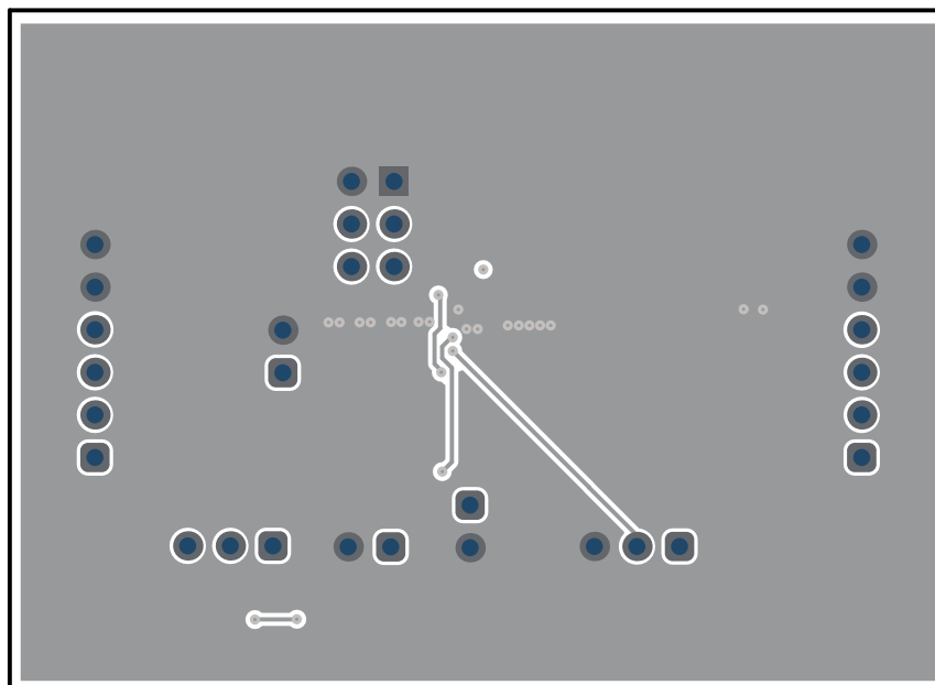
Figure 3-4. Bottom Layer
