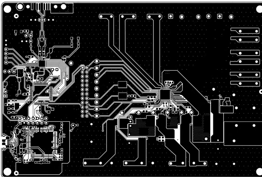
Figure 4-4. Top Layer
