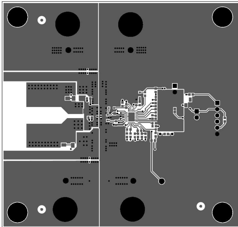
Figure 18. Bottom Layer
