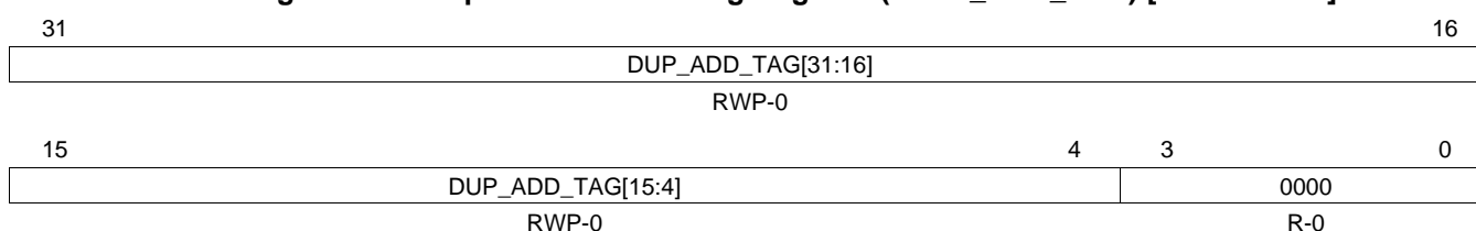
Figure 4-19. Duplicate Address Tag Register (FDUP_ADD_TAG) [offset = 2Ch]
