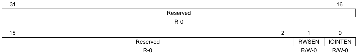
Figure 23-40. SDIO Interrupt Enable Register (SDIOIEN)
