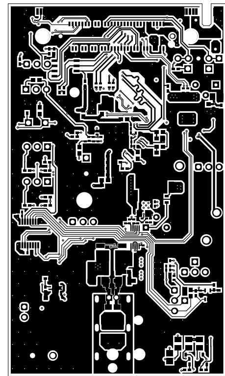
Bottom Layer
