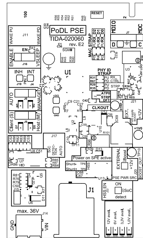
Top Overlay
